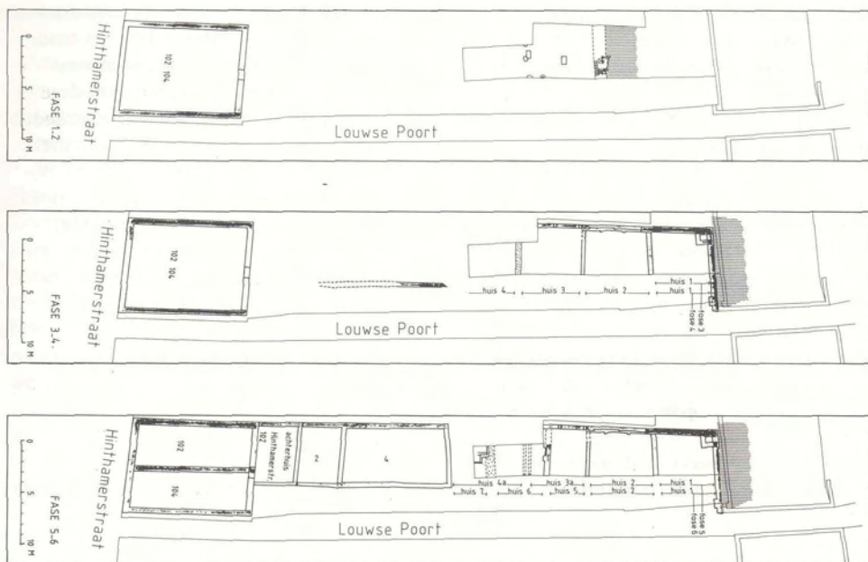
Afb. 4 De resultaten van het bouwhistorisch en archeologisch onderzoek en de opmetingsgegevens van het pand Louwse Poort 4; fase 1 1250-1300, fase 2 1275-1325, fase 3 1325-1350, fase 4 1350-1400, fase 5 1400-1450, fase 6 1450-1600 (Tekening BAD).
