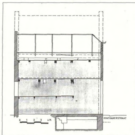
Afb. 2 Doorsnede Hinthamerstraat 104 en aanzicht van de rechterzijmuur (Tekening BAD).
